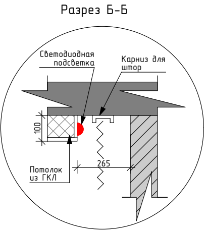
Пример монтажа
