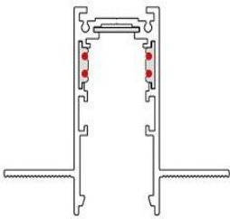
Разрез профиля от магнитно трековой системы.
